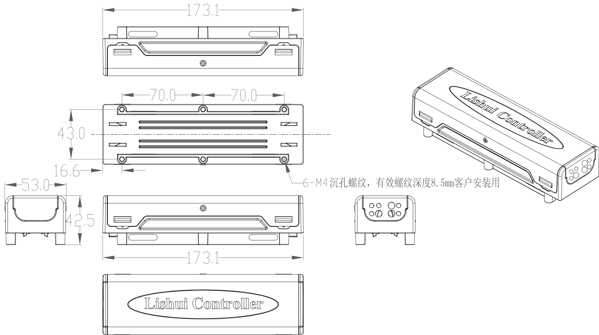
150Z_V05 外观图
